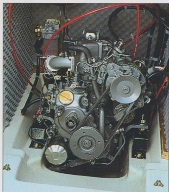
エンジン/コンパクトで力強い1GM-10Bを搭載。アウトボードタイプは9.9馬力対応とします。(写真はI/B-Sです)
